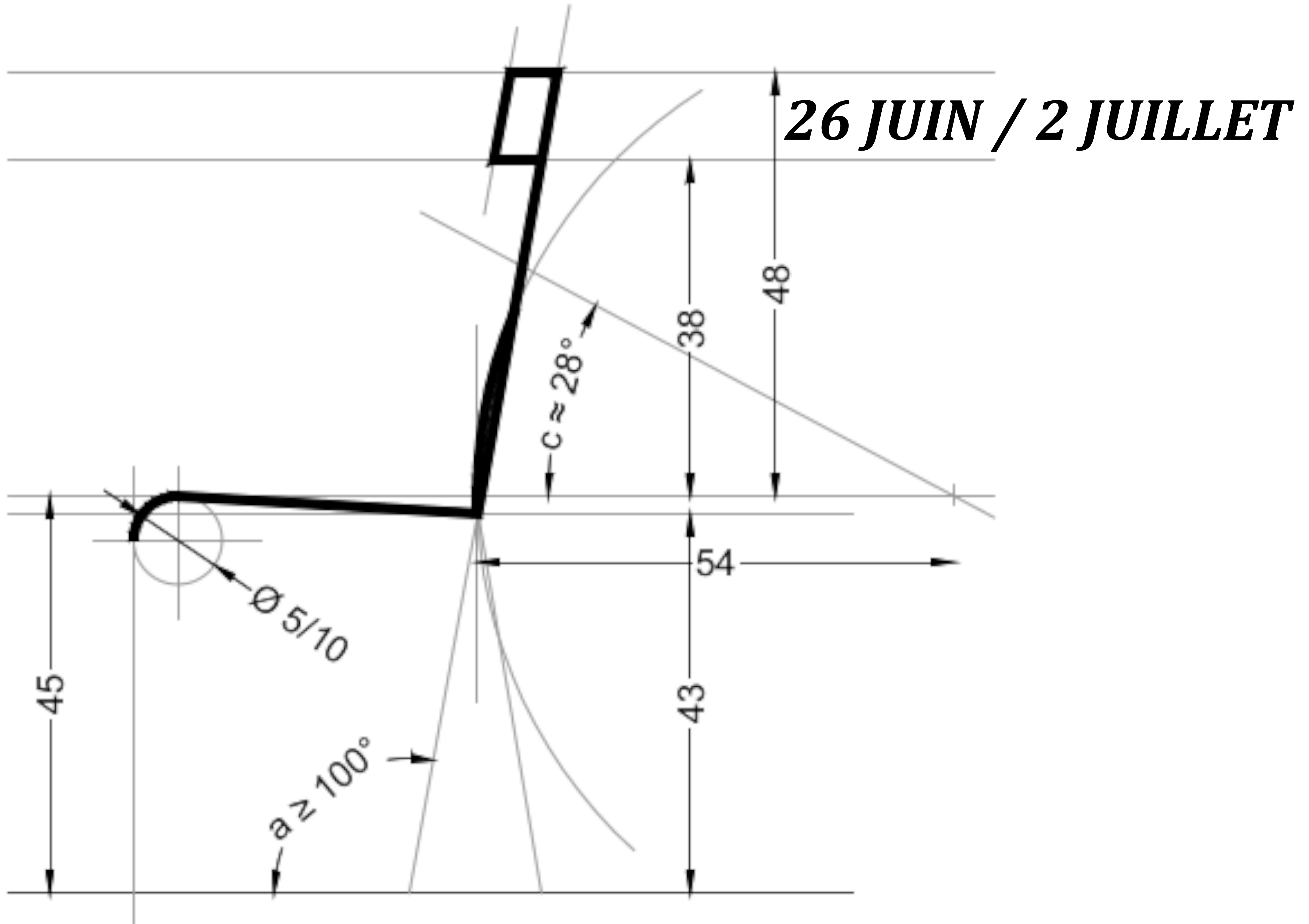
CHAISE profil & plan _ 1/2
